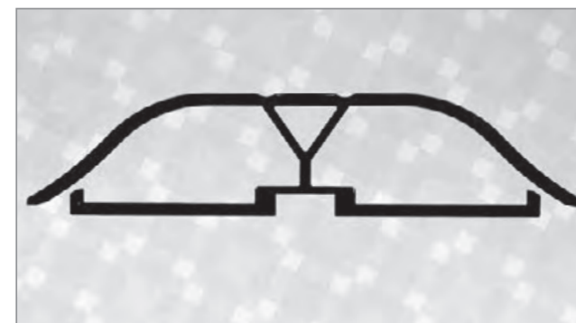
Querschnitt Profile
